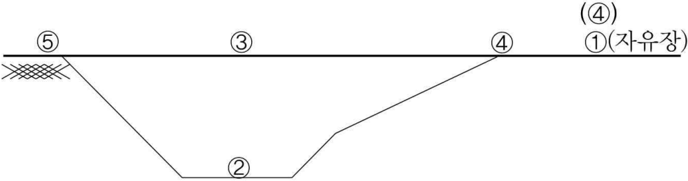
[별도 10] 기하학적 구조가 심하게 비대칭인 댐인 경우 지진가속도감지기 설치 위치 (제20조 관련)
